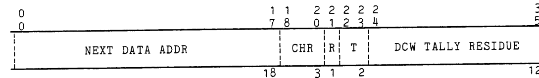
IOM Status Format
