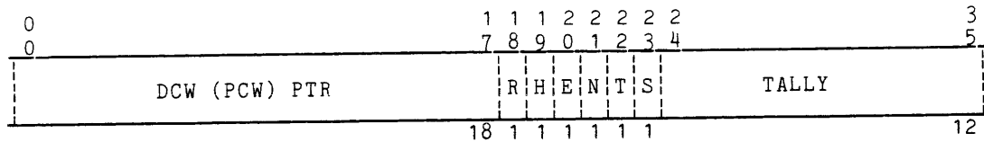
IOM LPW Format
