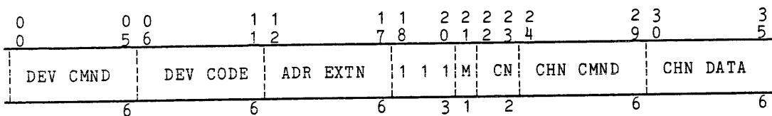
Figure 3-6. IOM Instruction DCW Format
