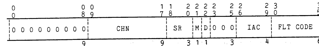
Figure B-1 (cont). IOM Formats
