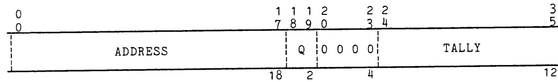
IOM SCW Format
