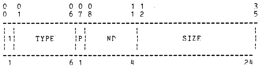
Figure 7-8. Argument Descriptor Format
