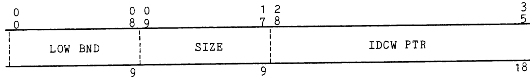
IOM LPW Extension Format
