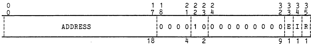
Figure 3-7. IOM Transfer DCW Format
