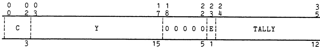
Figure 6-6. FNP IOM ICW Format
